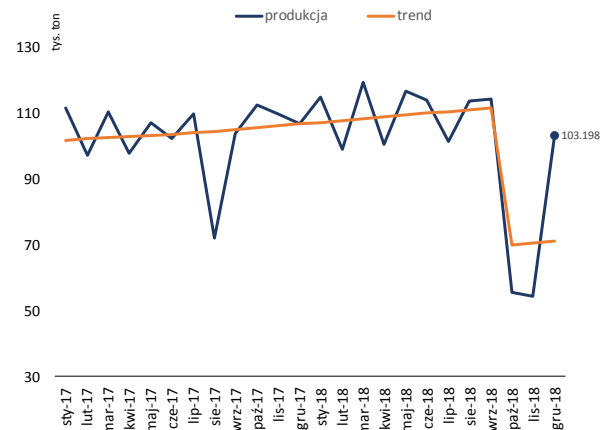
Wykres 16. Walcówka dane w tys. ton
