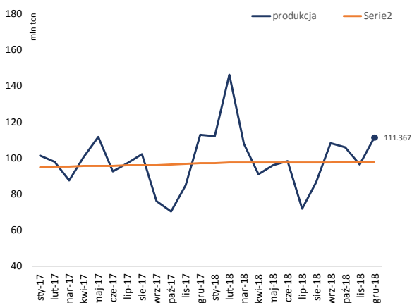
Wykres 15. Kształtowniki walcowane na gorąco dane w tys. ton
