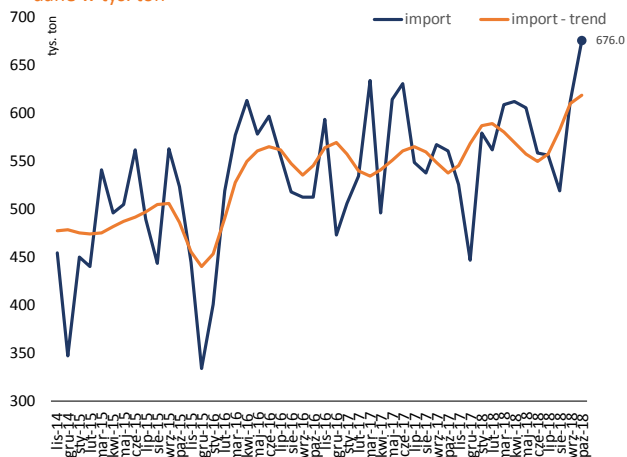
Wykres 21. Wyroby długie - import
