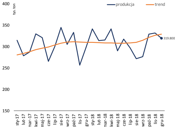
Wykres 13. Wyroby płaskie walcowane na gorąco dane w tys. ton
